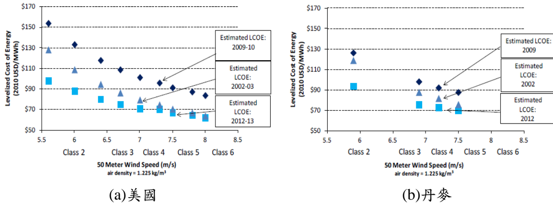
圖9、NREL評估2002~2013年美國與丹麥在不同級數之風力發電成本[6]
