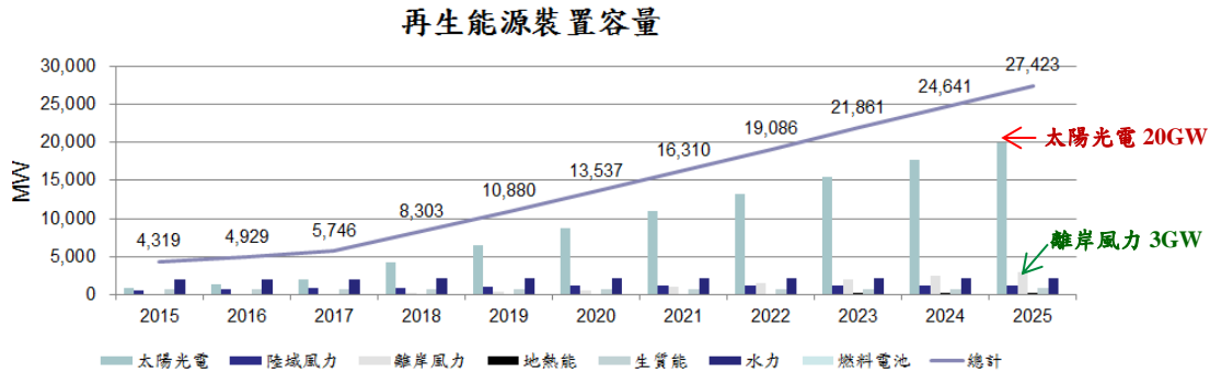
圖14、2016年5月經濟部提出2025年再生能源發電占總發電量20%
