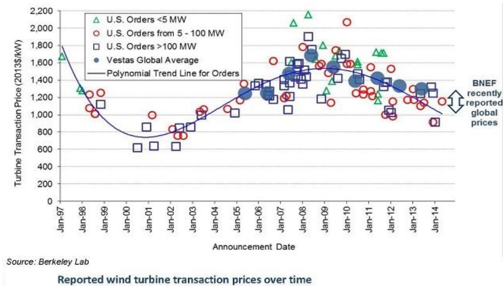
圖 11、美國的風力發電機組交易價格[14]
