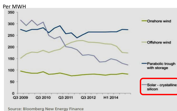
圖 8、FS-UNEP 之太陽光電與風力發電均化成本變化趨勢[10]
