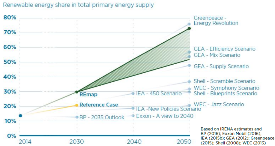
圖2、未來全球再生能源占比趨勢[3]
