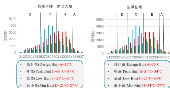
圖 19 建築負載區間
