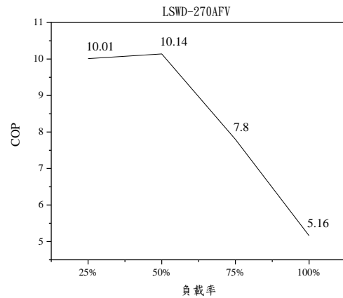
圖 13 A 型螺旋式冰水機實際測量數據
