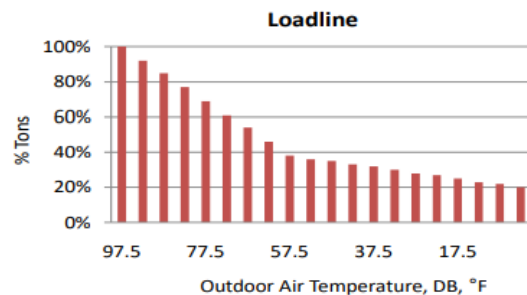
圖 14 冰水機負載曲線圖[9]
